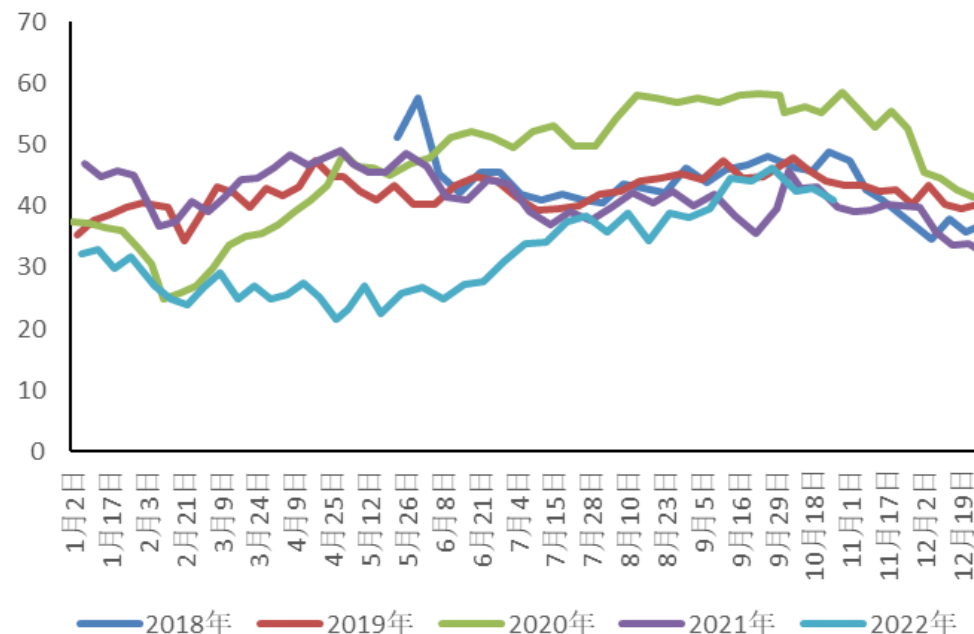
开工率:石油沥青装置 (%)
