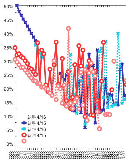
图24: 2021-07月期权合约隐含波动率结构分布
