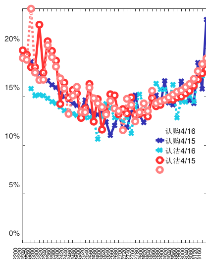
图23: 2021-09月期权合约隐含波动率结构分布
