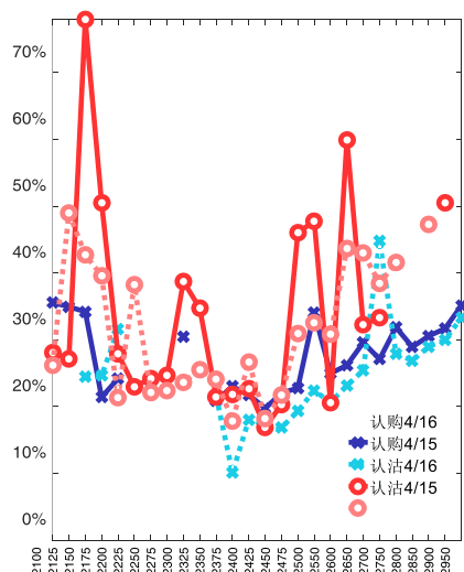
图191：2021-06月期权合约隐含波动率结构分布
