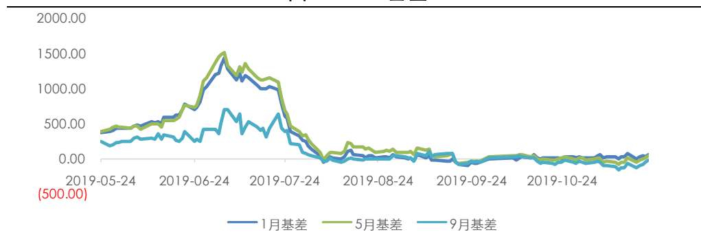
图 1：PTA 基差
