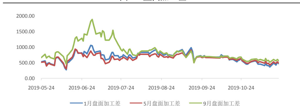
图 3：盘面加工差
