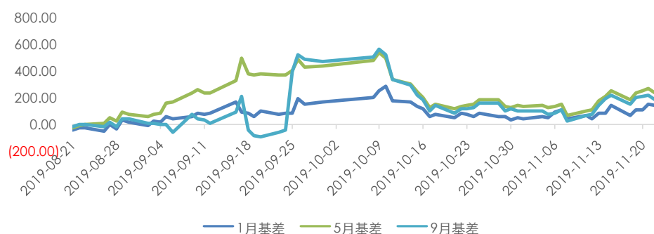
图 7：MEG 基差
