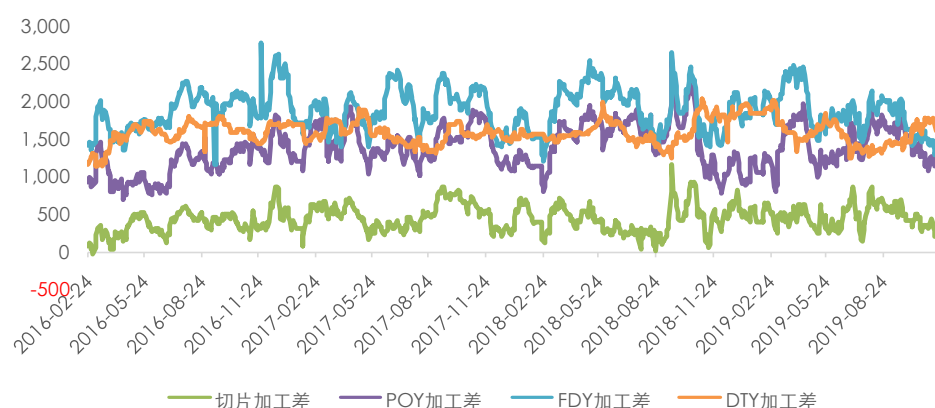
图 13: POY、FDY、DTY 加工差
