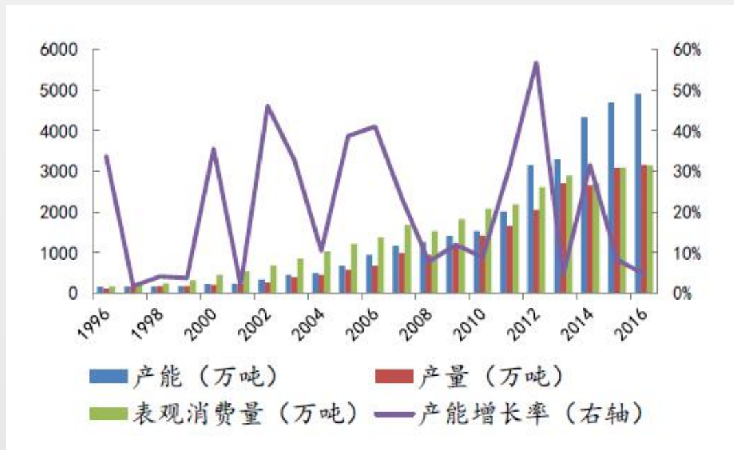
我国PTA产能、产量、消费及增长率情况图
